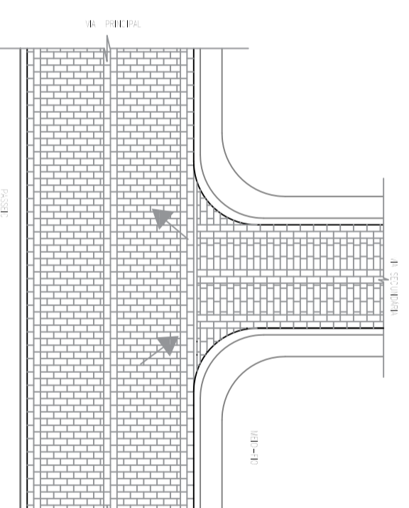
ASSENTAMENTO NOS ENTROCAMENTOS
