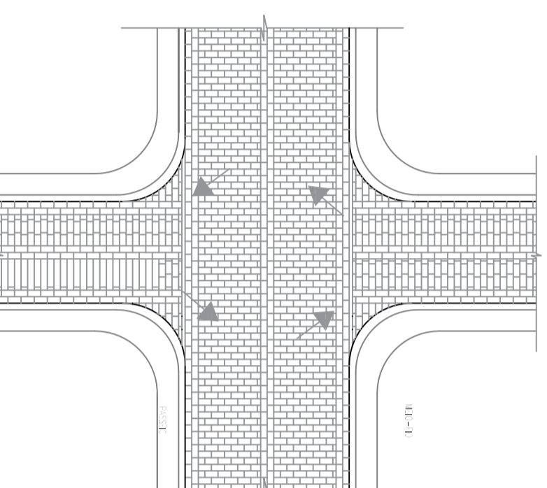
ASSENTAMENTO NOS CRUZAMENTOS RETOS
