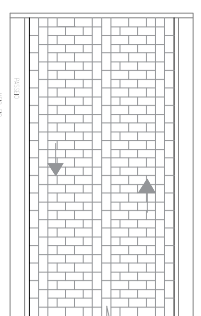
CASO NORMAL DE ASSENTAMENTO DE PARALELEPÍEDOS
