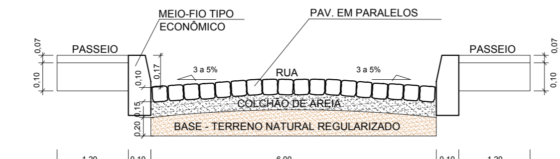
SEÇÃO TRANSVERSAL TIPO - DETALHE S / ESCALA
