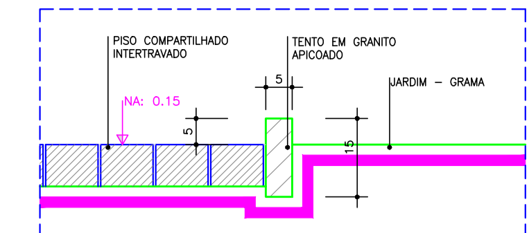
DET. TÍPICO CANTEIROS ESCALA 1/10
