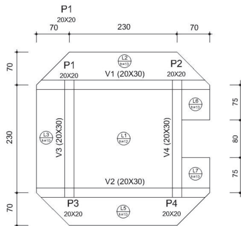
PLANTA DE FORMA - VIGA E LAJE SUPERIOR
