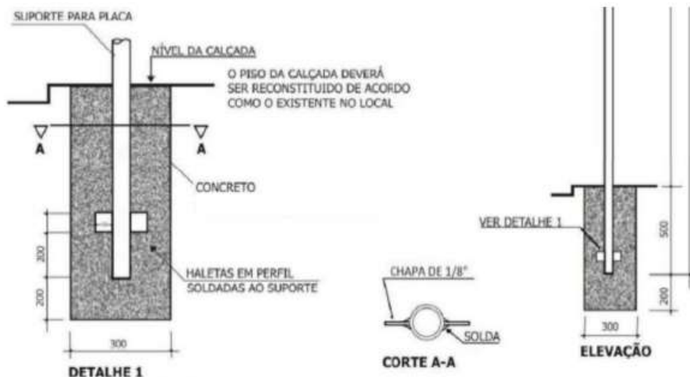
Figura 2 – Detalhe do dispositivo antigo e da fundação.
