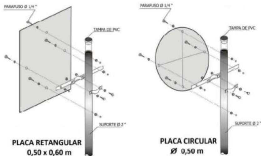
Figura 1 – Detalhe de fixação das placas.
