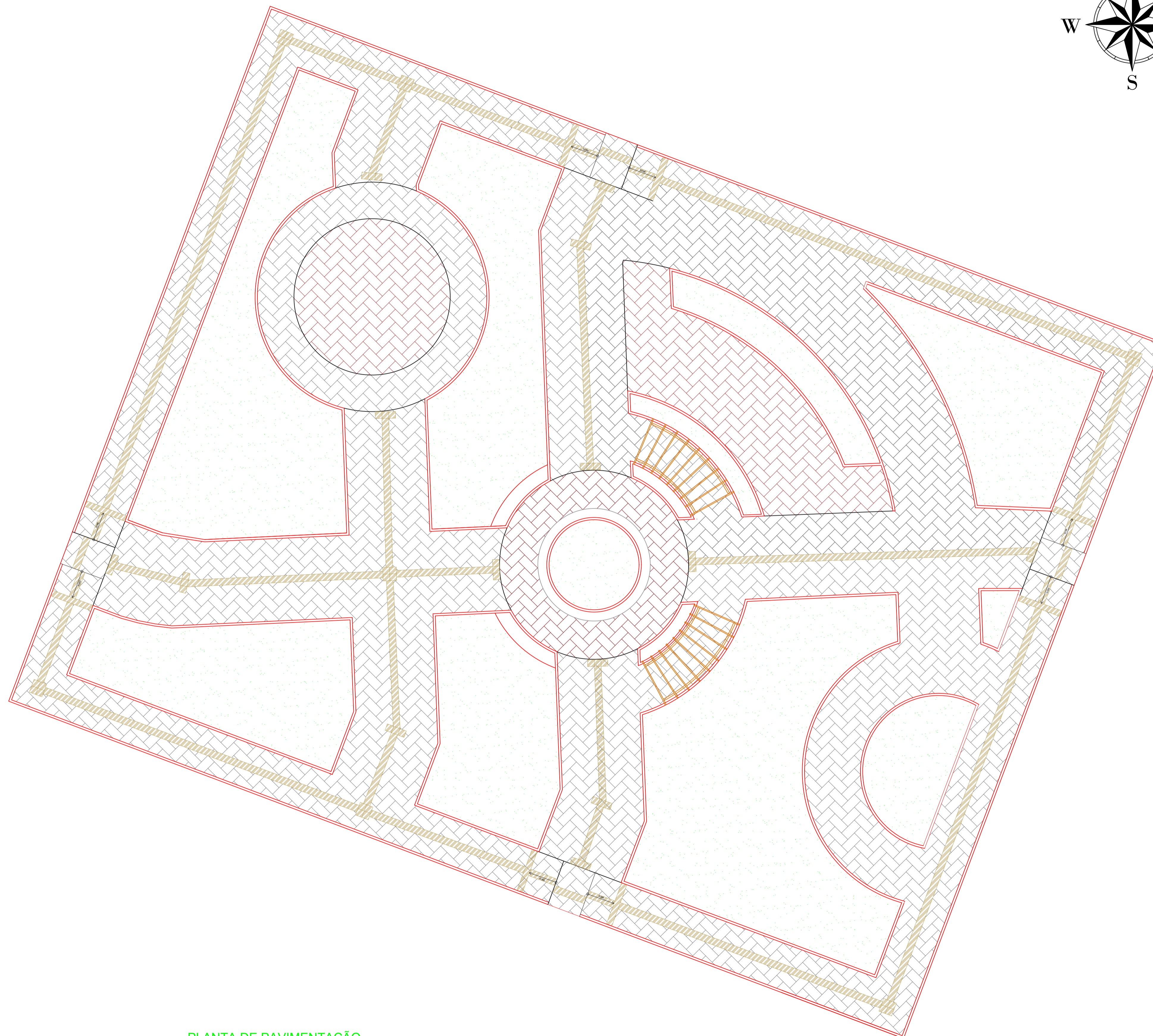
PLANTA DE PAVIMENTAÇÃO ESCALA 1/100
