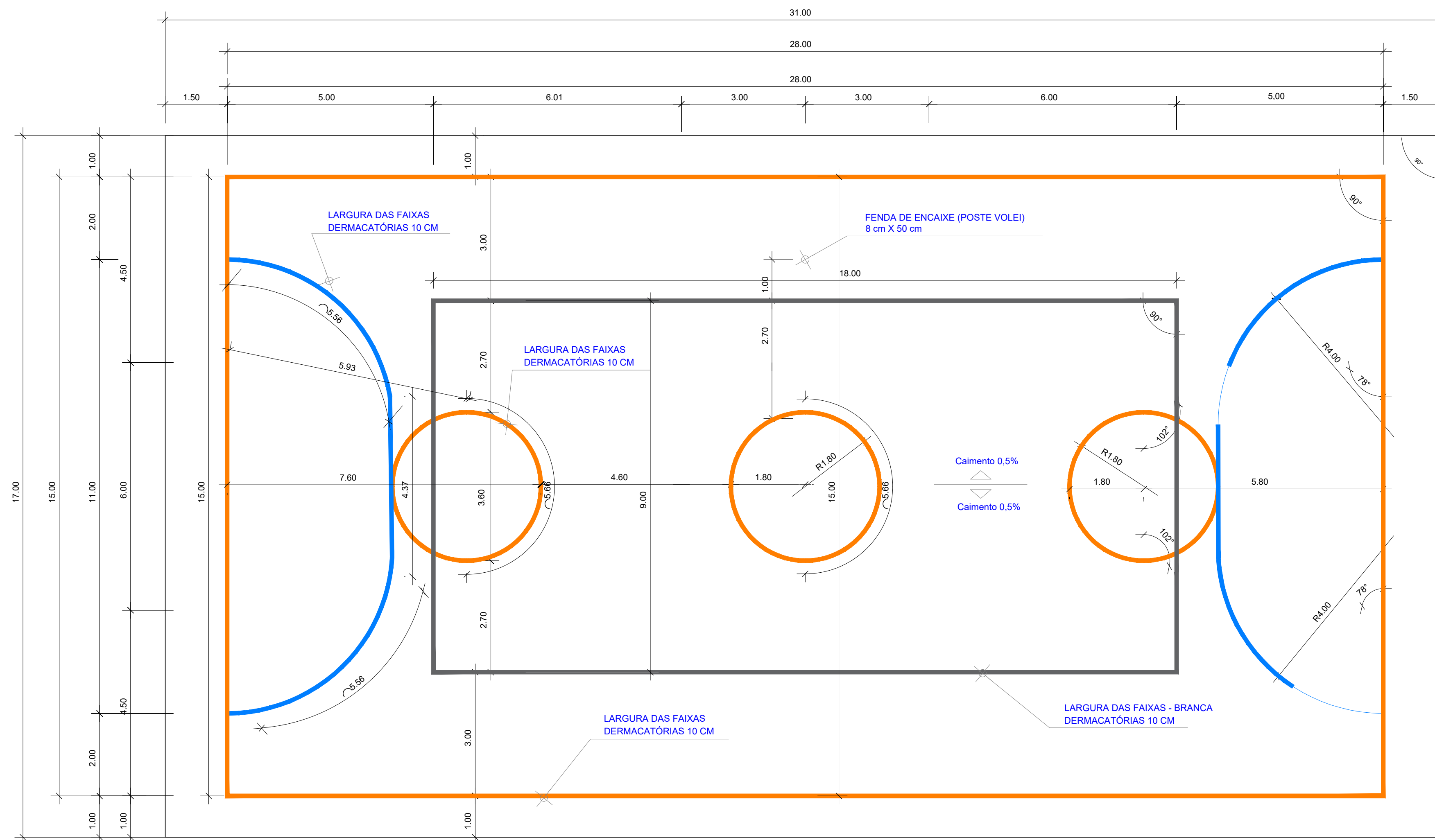
Planta Baixa - Quadra Escala 1/75
